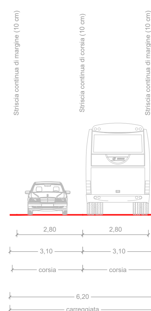
Tipico Viabilità - Stato futuro scala 1:100
