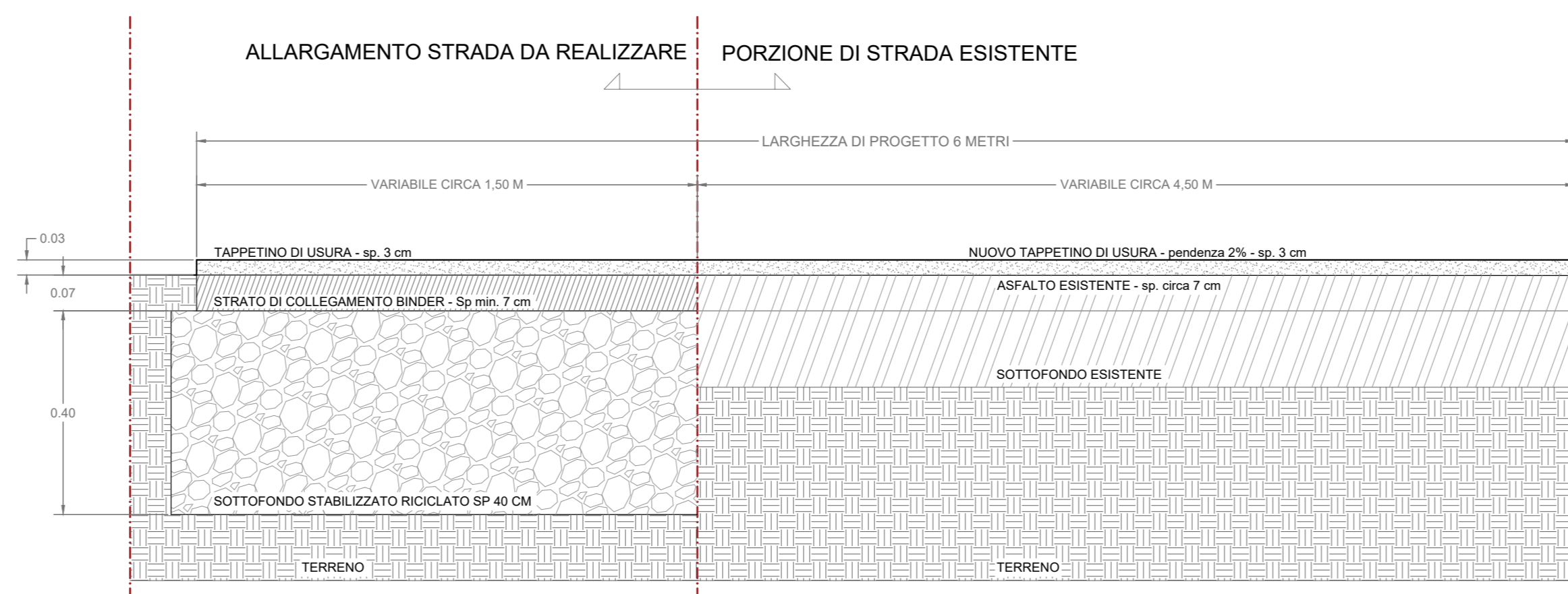
Tipico Stratigrafia - Stato futuro scala 1:10
